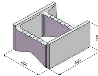
KB Z-40 RAPID průběžná objem dutin v m 3 0,03424
