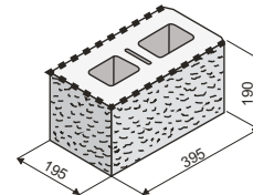
KB 11-21 B objem dutin v m 3 0,00416
