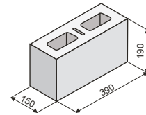
KB 1-15 A děl. objem dutin v m 3 0,00476
