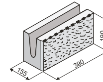
KB 101-15 B objem dutin v m 3 0,003272
