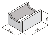
KB Z-30 objem dutin v m 3 0,0159
