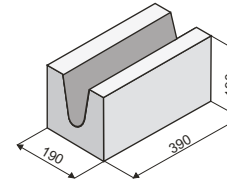
KB 101-20 A objem dutin v m 3 0,00397
