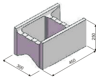
KB Z-30 RAPID průběžná objem dutin v m 3 0,02412
