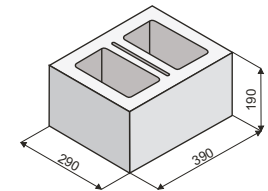
KB 1-30 A objem dutin v m 3 0,0123
