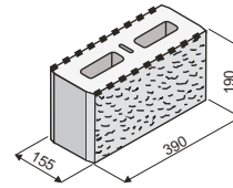
KB 7-15 B objem dutin v m 3 0,00238
