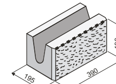
KB 101-21 B objem dutin v m 3 0,00424
