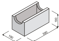
KB Z-20 objem dutin v m 3 0,0089
