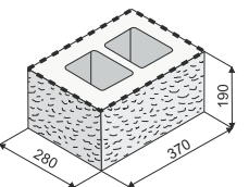
KB 15-21 B objem dutin v m 3 0,00737
