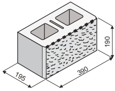
KB 1-21 B objem dutin v m 3 0,00596
