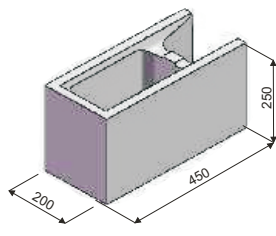
KB Z-20 RAPID koncová objem dutin v m 3 0,01375
