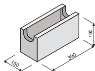
KB Z-15 objem dutin v m 3 0,0062
