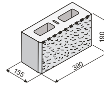
KB 1-15 B objem dutin v m 3 0,00342
