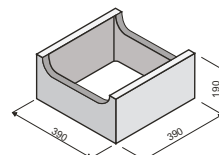
KB Z-40 objem dutin v m 3 0,0228
