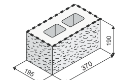
KB 13-21 B objem dutin v m 3 0,00365
