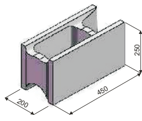
KB Z-20 RAPID průběžná objem dutin v m 3 0,01409
