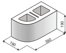
KB 6-20 A objem dutin v m 3 0,00676
