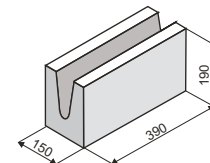
KB 101-15 A objem dutin v m 3 0,00336
