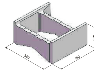
KB Z-50 RAPID průběžná objem dutin v m 3 0,04435
