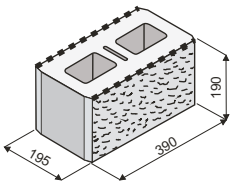
KB 7-21 B objem dutin v m 3 0,00459
