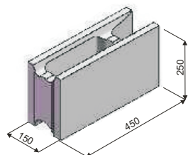
KB Z-15 RAPID průběžná objem dutin v m 3 0,00886
