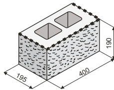
KB 9-21 B objem dutin v m 3 0,00574
