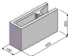
KB Z-15 RAPID koncová objem dutin v m 3 0,00869
