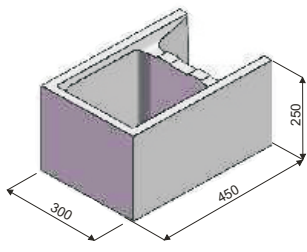
KB Z-30 RAPID koncová objem dutin v m 3 0,02364
