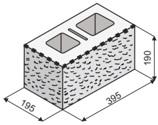
KB 5-21 B objem dutin v m 3 0,0055
