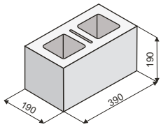
KB 1-20 A děl. objem dutin v m 3 0,00692
