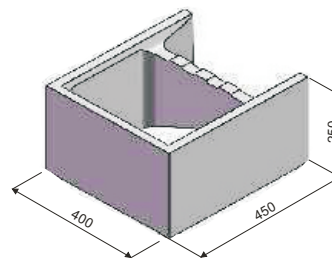
KB Z-40 RAPID koncová objem dutin v m 3 0,03357
