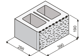
KB 1-31 B objem dutin v m 3 0,01098
