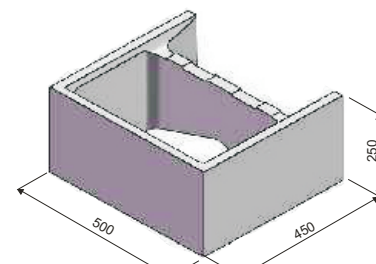
KB Z-50 RAPID koncová objem dutin v m 3 0,04350
