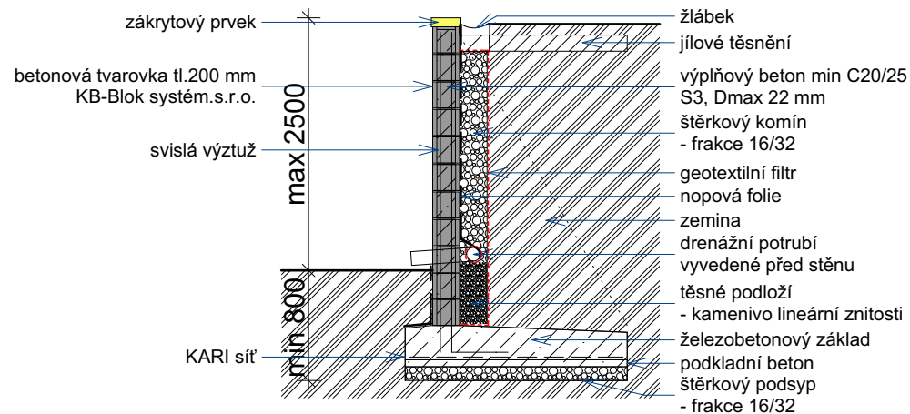
Schematická řez - odvodnění základové spáry před opěrnou stěnu
