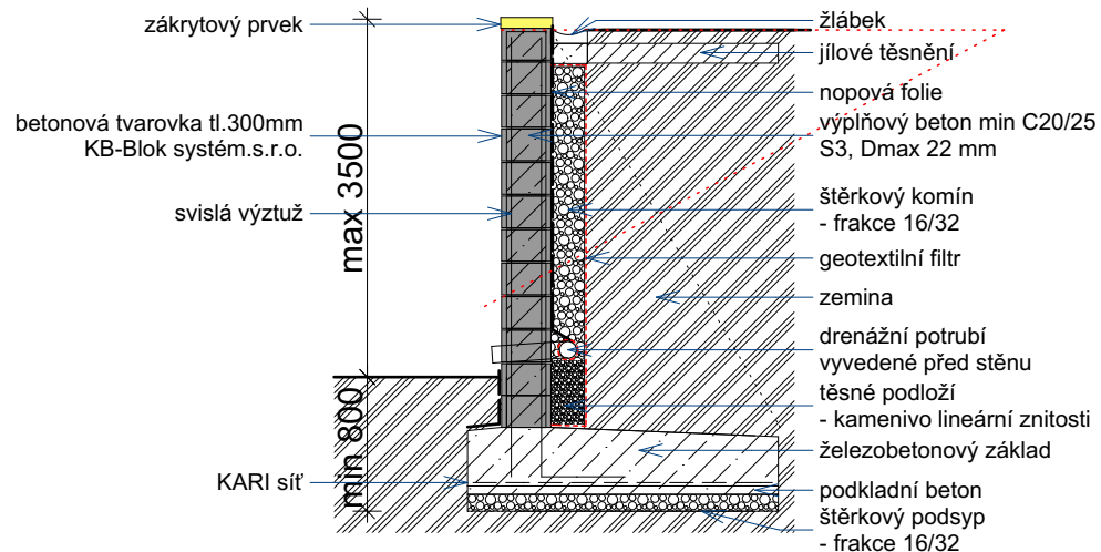
Schematická řez - odvodnění základové spáry před opěrnou stěnu
