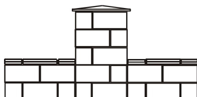
Rozměr : 60 x 60 cm Použití tvarovky : KB 6-20 A
